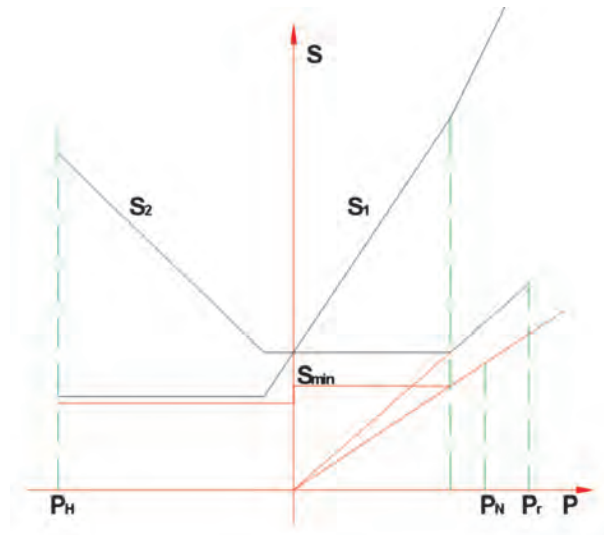
Rys. 2. Napinanie nadążne z modułem stałonapięciowym
